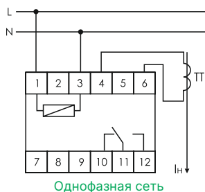
Однофазная сеть
