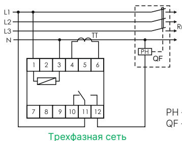
Трехфазная сеть
