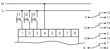
8-7-6 – контакт мгновенного действия.
