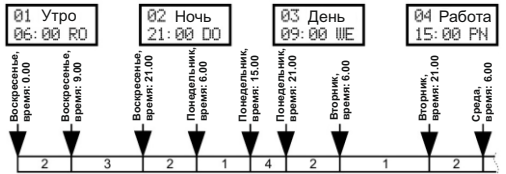
Выполнение программ
